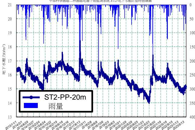
中部科學園區二林園區地層下陷監測系統 ST2-地下水壓計歷時曲線圖
